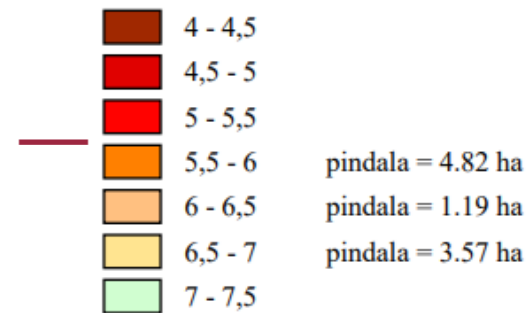
Mullareaktsiooni kaart pH
