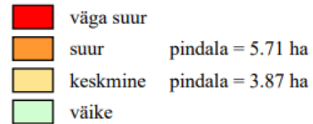
K (mg/kg) väetustarve kaart
