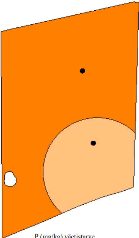
P (mg/kg) väetistarve
