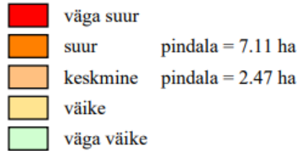
P (mg/kg) väetistarve
