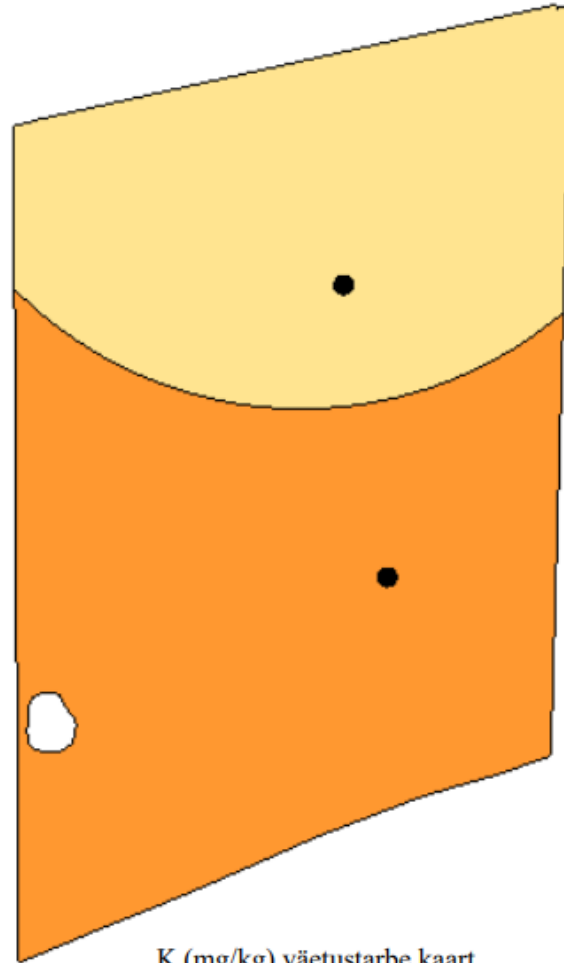
K (mg/kg) väetustarve kaart
